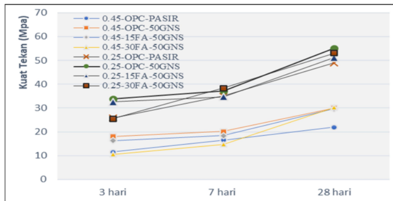
Gambar 5. Hubungan kuat tekan dengan umur beton
